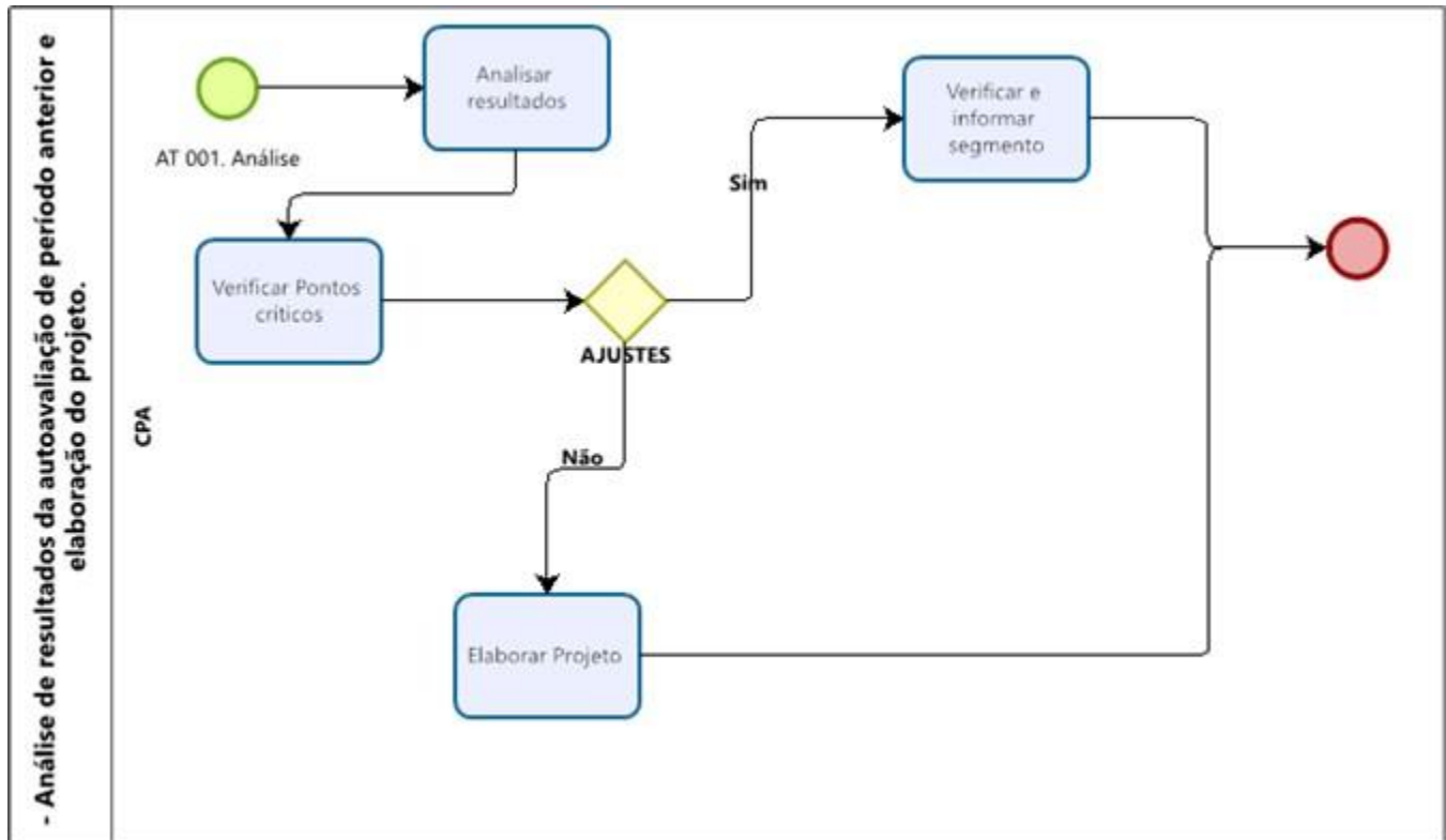
Figura 2. Primeiro processo executado pela CPA quando inicia o ano / período, o de análise de resultados da autoavaliação do ano anterior.
